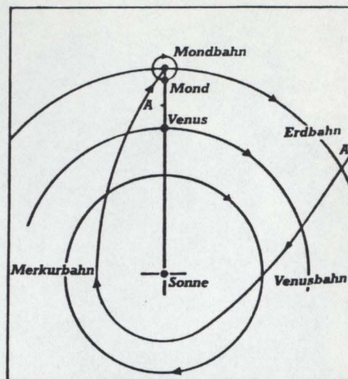
Den kosmiska konstellationen den 5. juni 8498 f Kr: Asteroiden (A) påverkas av dragningskraften, vilken orsakas av den trefaldiga konstellationen av solen, Venus, månen och jorden, och kastas ur sin bana. I sin nyvunna bana störtar den nu i kollisionskurs mot jorden.
