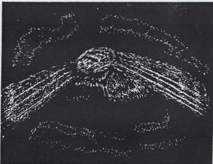
© Ovanligt norrskenfenomen över Karlskoga. Ungefär så här såg det ut vid ett tillfälle på natten omkring kl. 03.45 den 13 april 1981 (se artikeln). Det är naturligtvis väldigt svårt att med pennan återge skådespelet, men här ett tappert försök.
